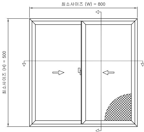
230SL - 이중창 ELEVATION (INSIDE VIEW - 내관도 : A-TYPE)
