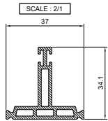
(단열공정취부)
