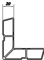
MUL0013016 THK 1.5 1.462 kg/m (VENT용)
