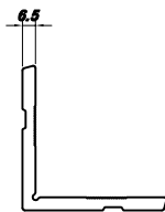
035PJ19115 ★ THK 6.5 2.263 kg/m (VENT FRAME용)
